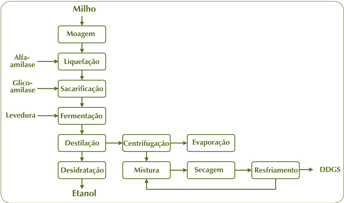
Figura 14 – Diagrama de fluxo do processo via seca para a produção de bioetanol de milho
