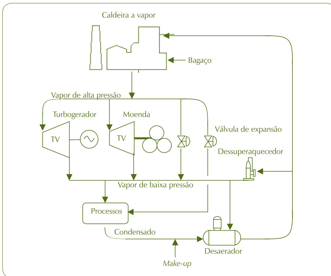
Figura 18 – Configuração usual do sistema de co-geração na agroindústria canavieira
