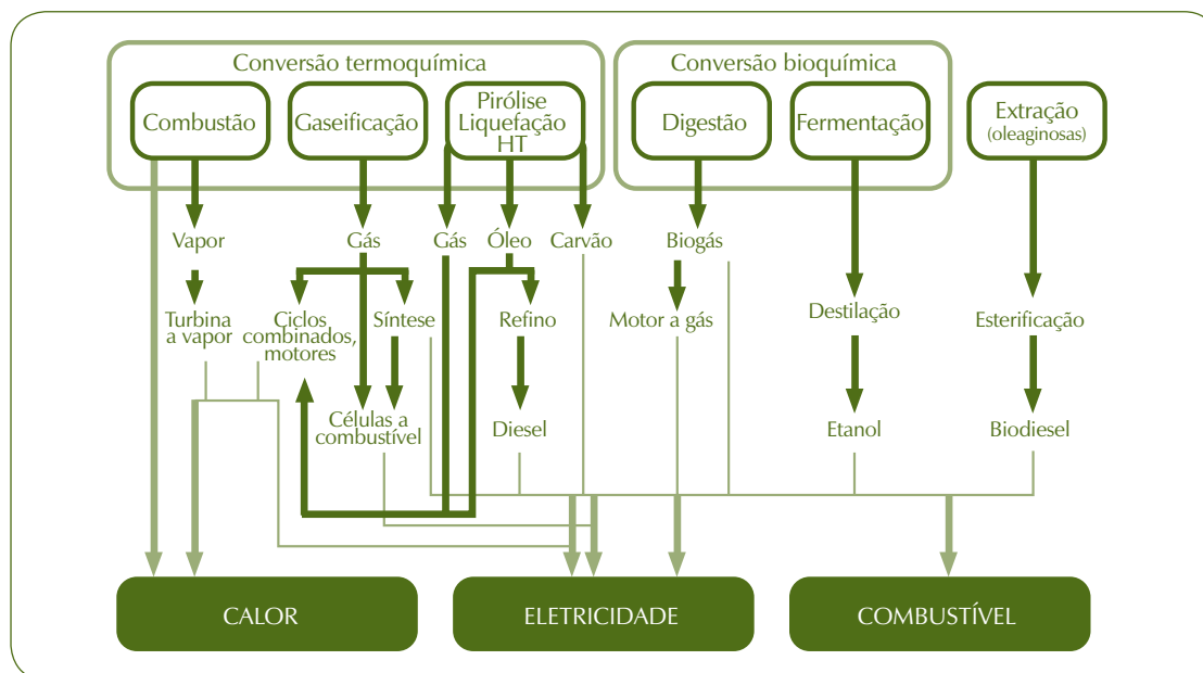
Figura 3 – Rotas tecnológicas para produção de bioenergia
