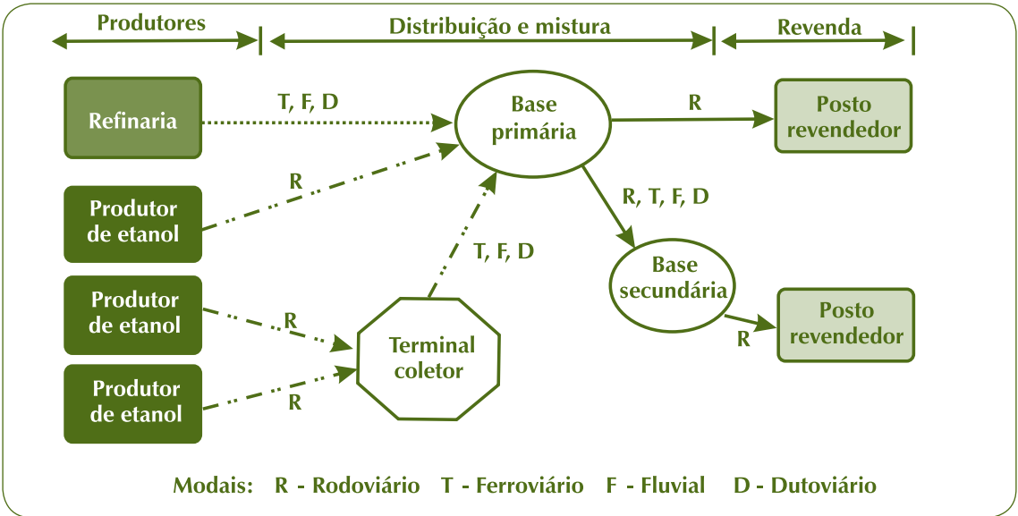
Figura 6 – Logística da gasolina e do etanol no Brasil
