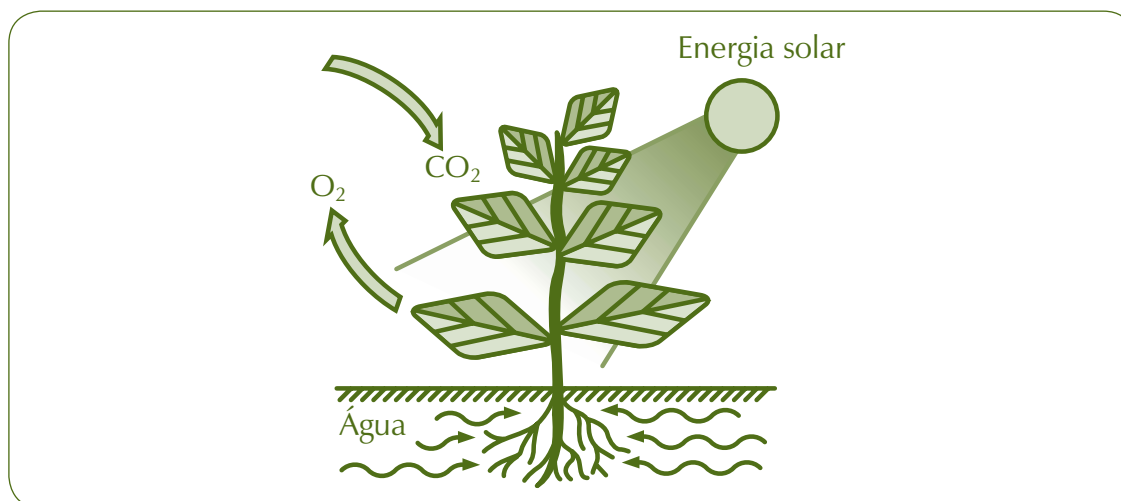
Figura 1 – O processo de fotossíntese
