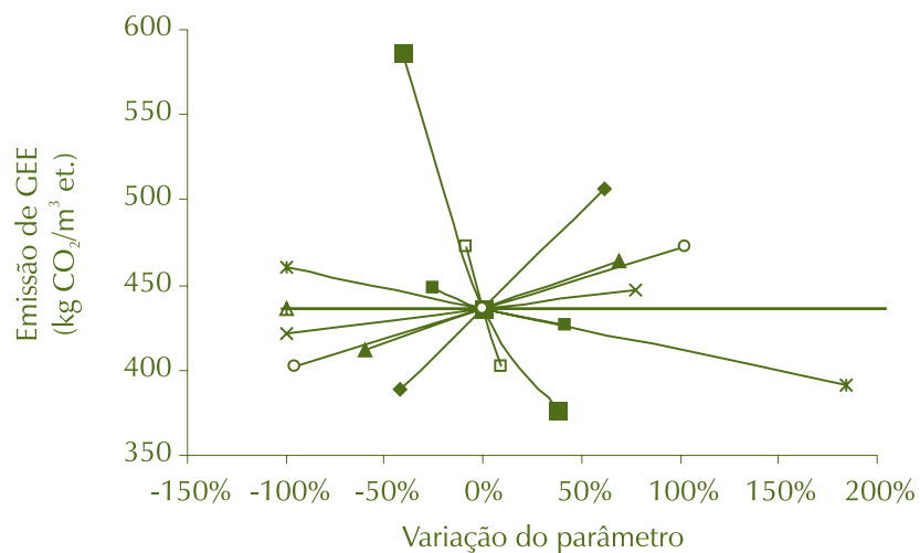
Figura 17 – Análise de sensibilidade para as emissões de GEE para o bioetanol de cana-de-açúcar no cenário atual (2005/2006)
